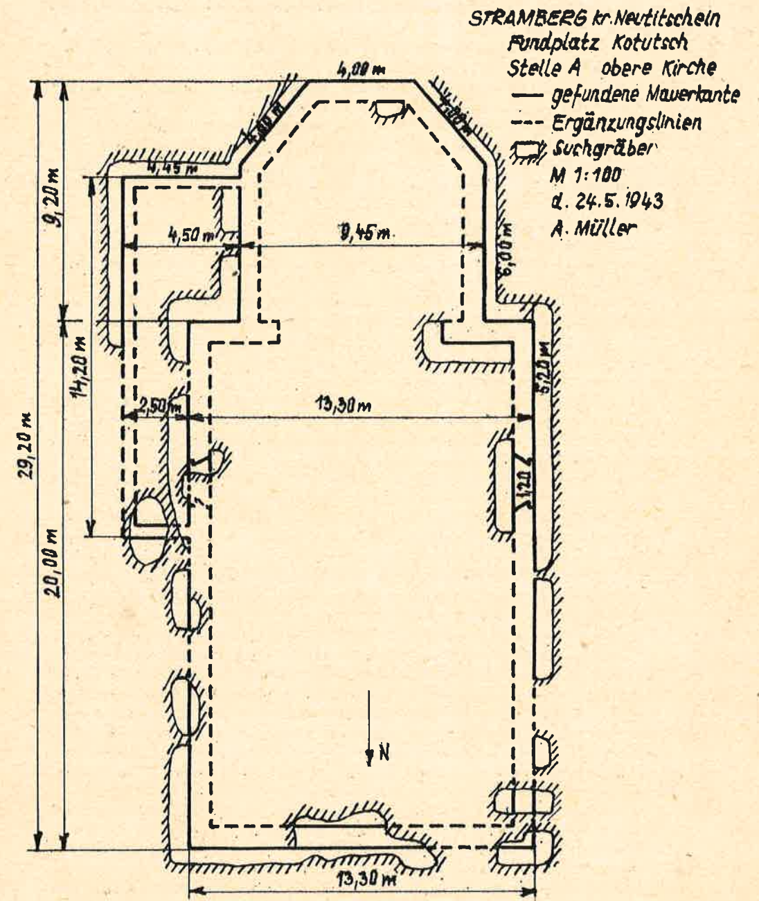
Plánek horního kostela pořízený A. Müllerem 24. 5. 1943 v měřítku 1:100, Reprodukce plánu 1:200.
