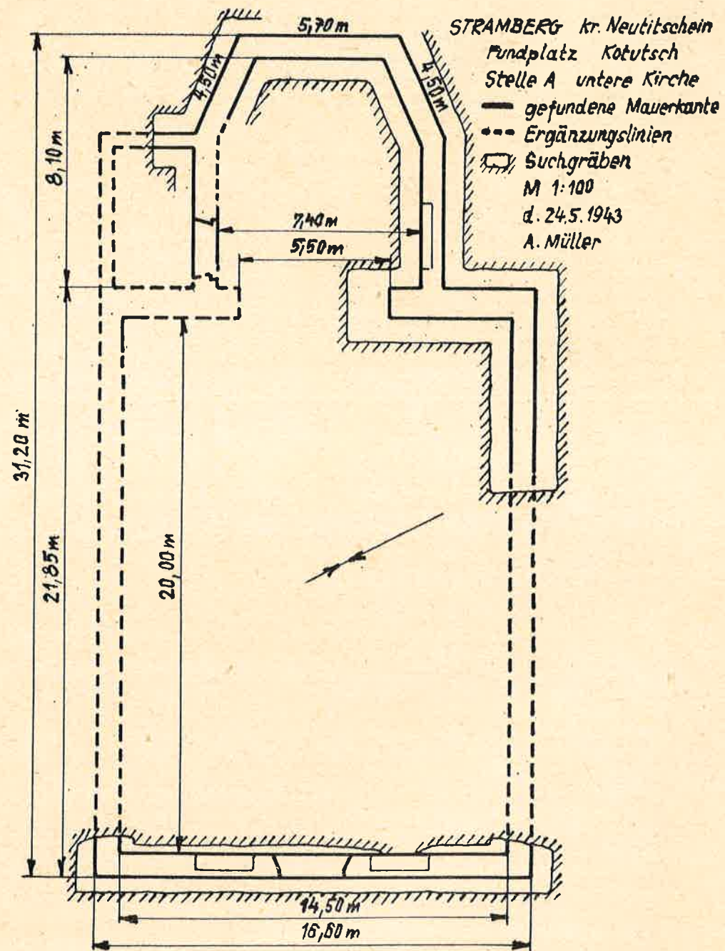
Plánek dolního kostela pořízený A. Müllerem 24. 5. 1943 v měřítku 1:100, Reprodukce plánu 1:200.
